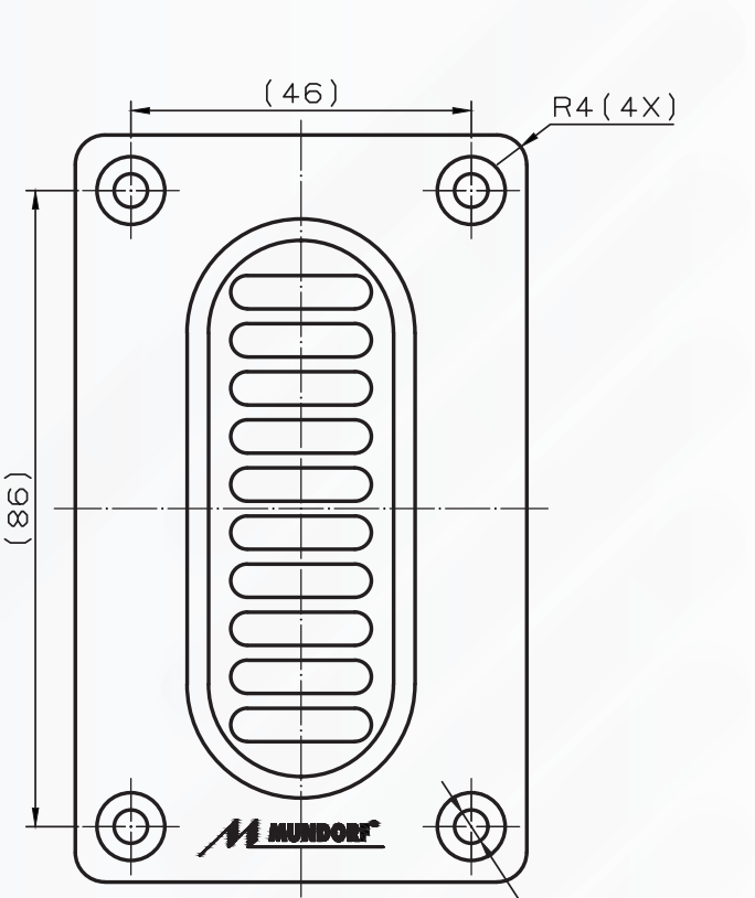
Ansicht Vorne
