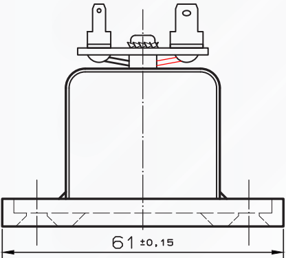
Draufsicht
