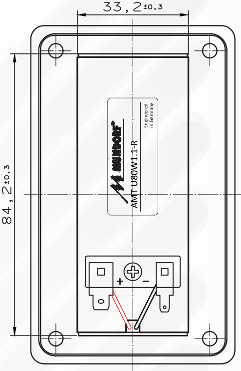
Ansicht Hinten
