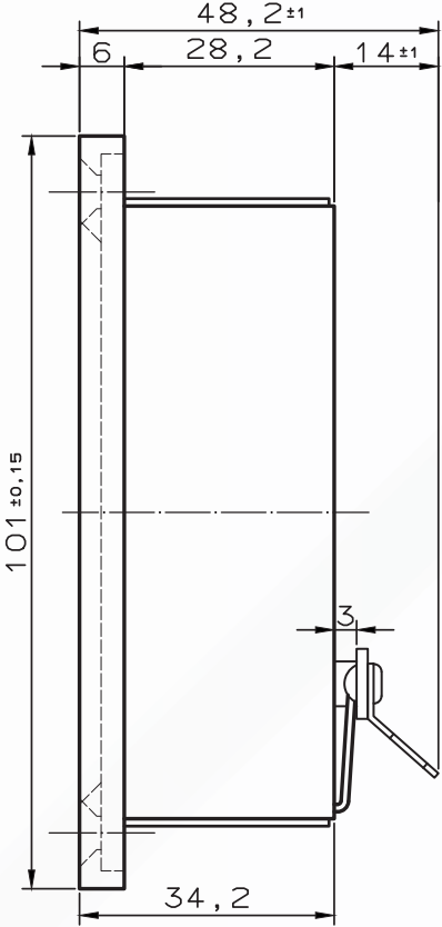
Seitenansicht
